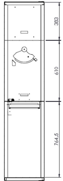
SEZIONE A-A
