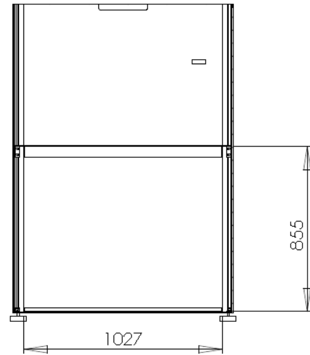
SEZIONE B-B
